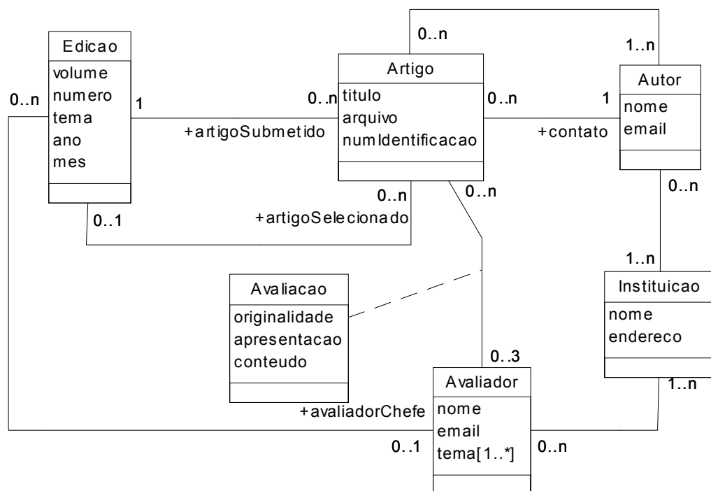
Figura 2 – Diagrama de Classes de Análise: Controle Edição.
