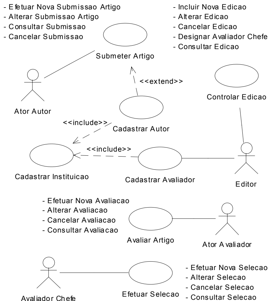
Figura 1 – Diagrama de Casos de Uso: Controle Edição.
