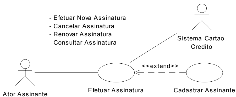
Figura 3 – Diagrama de Casos de Uso: Assinatura.
