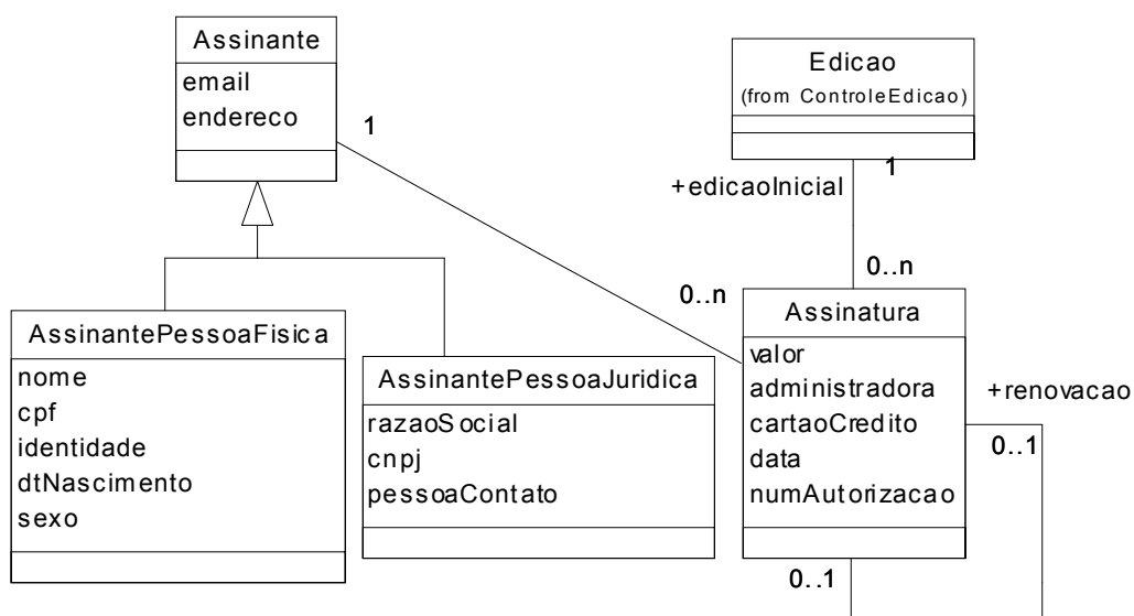
Figura 4 – Diagrama de Classes de Análise: Assinatura.
